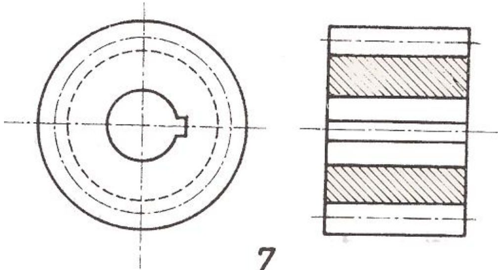
Dişli, m=4 , z=12 , 2 adet
