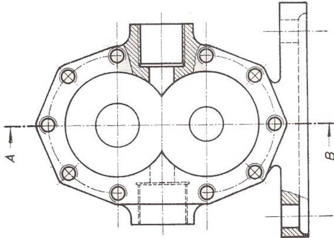
Gövde
