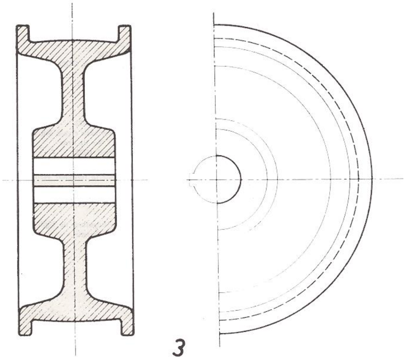
Kasnak
