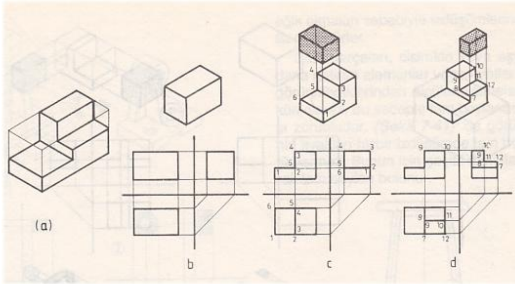
Önden görünüşün elde edilmesi.
