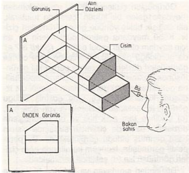
Önden görünüşün elde edilmesi.
