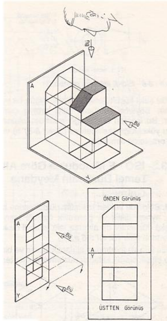
Üstten görünüşün elde edilmesi.
