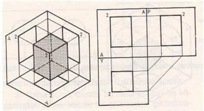
Önden görünüşün elde edilmesi.
